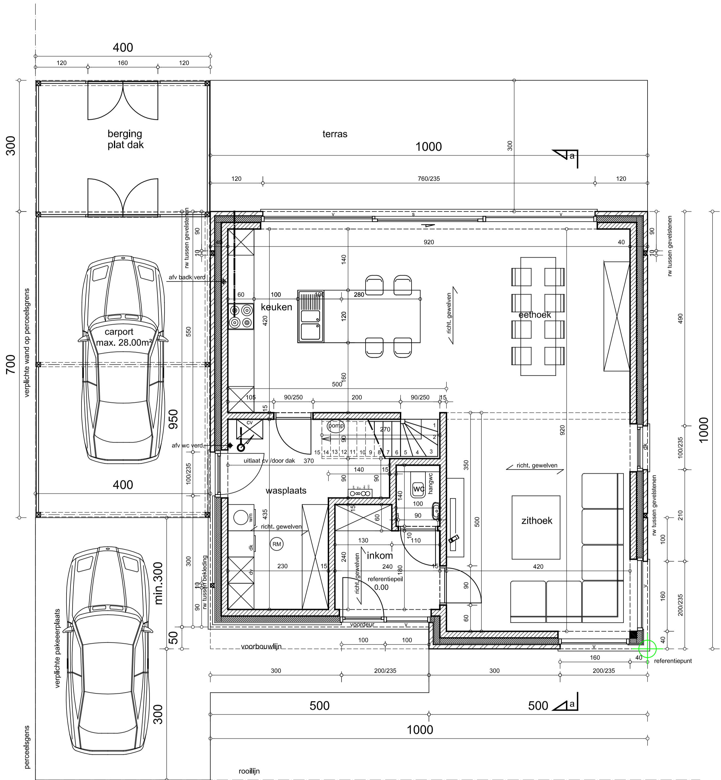
gelijkvloers / 1:50
